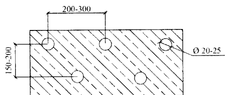
Расположение шпуров
